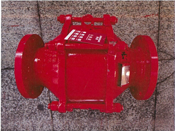
图 1. 阻火器
